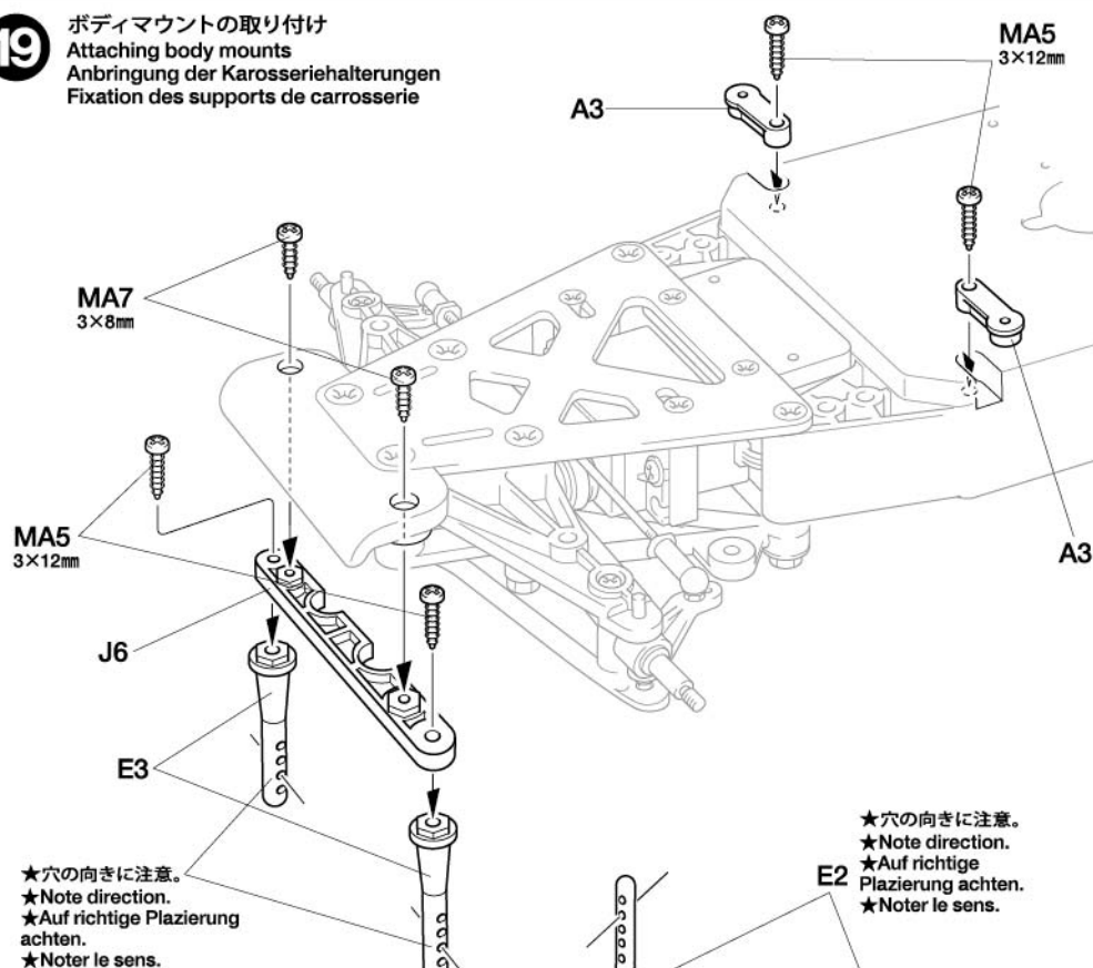
MA5 x6 3×12mmタッピングビス Tapping screw Schneidschraube Vis taraudeuse
