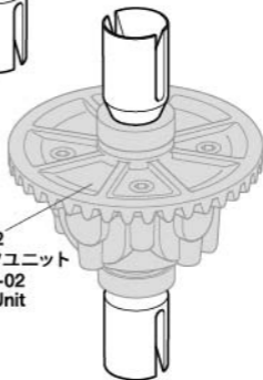
※デフジョイントカップ ※Differential cup joint
