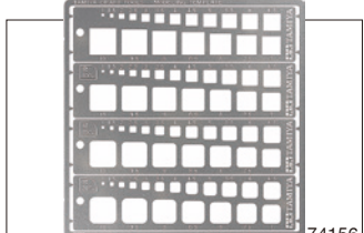
モデリングテンプレート(正方形1~10mm) 74156
